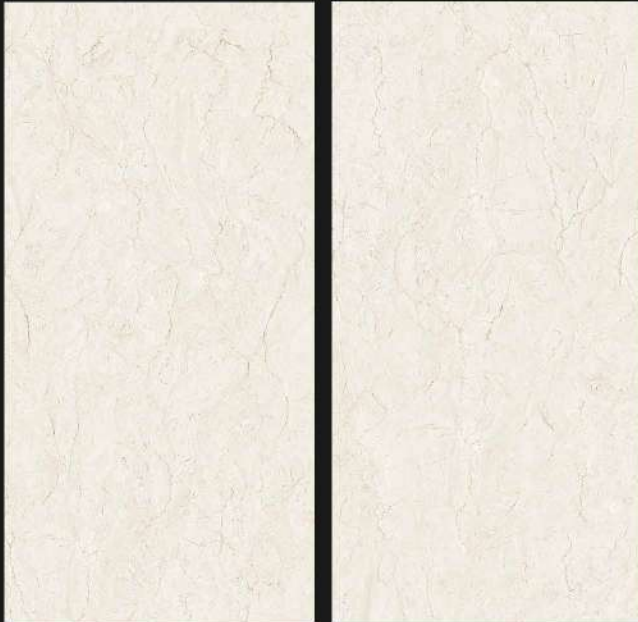
CANFIS
